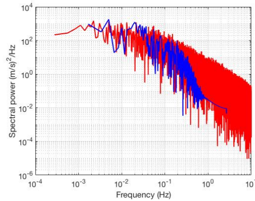
(d) Power spectral density at R = 20 km
